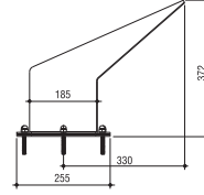
Yandan görünüş
