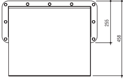
Üstten görünüş
