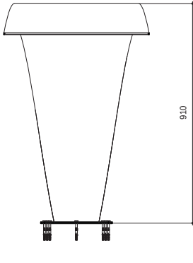
Önden görünüş
