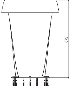
Önden görünüş
